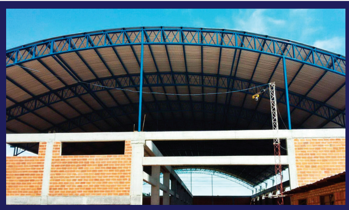
PROVINDUS S.A (CAPIATÁ) ESTRUCTURA DE FORMA PARABÓLICA.
